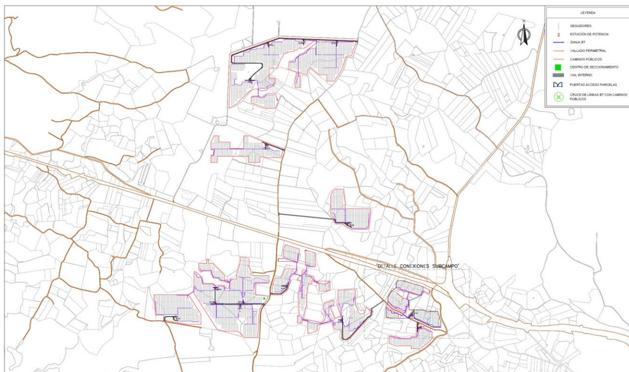
Ilustración 4. Líneas de baja tensión de la versión actual del proyecto
