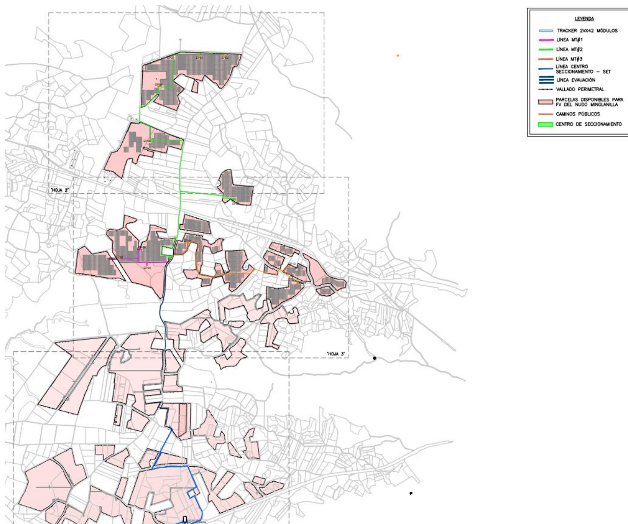
Ilustración 3. Líneas de media tensión de la versión anterior del proyecto
