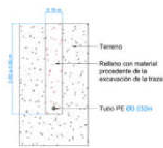
Figura 5. Esquema de microzanja
