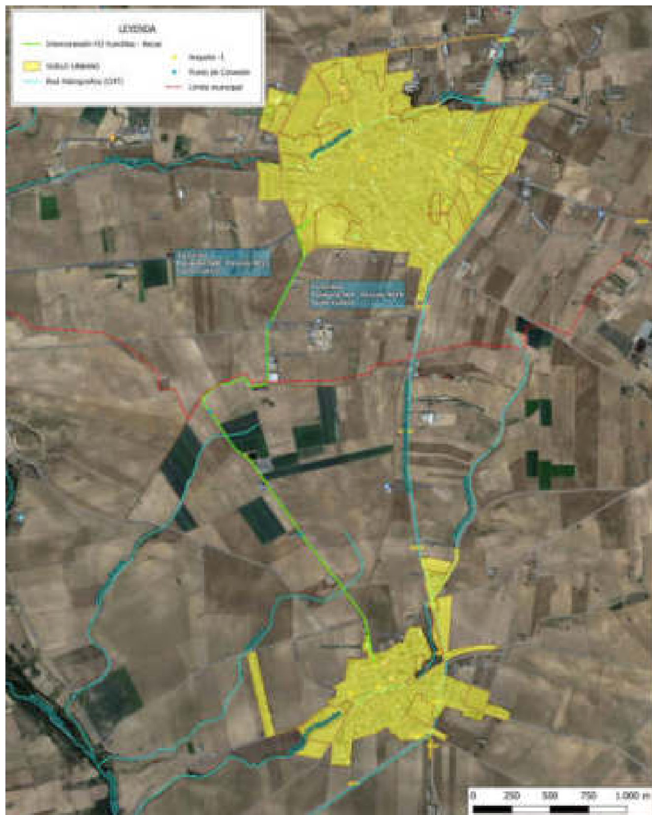
Figura 1. Trazado de la instalación en ambos términos municipales.
