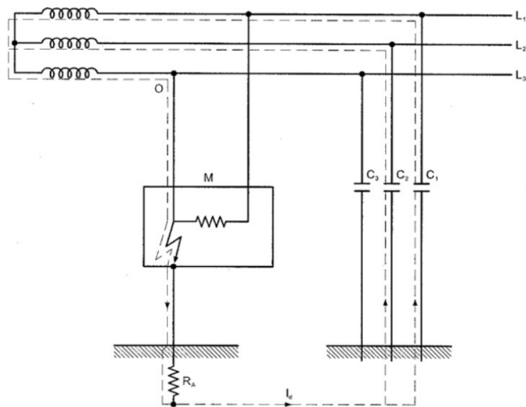
Figura 6.1. Esquema IT aislado de tierra
