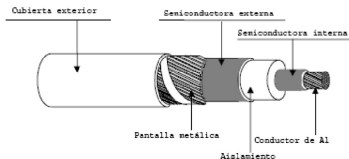
Imagen 1. Componentes del conductor de alta tensión
