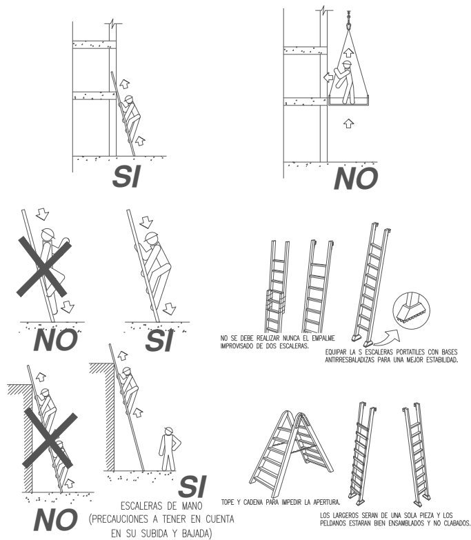
POSICION CORRECTA DE ESCALERAS DE MANO POSICIONES INCORRECTAS DE ESCALERAS DE MANO
