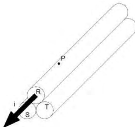
Figura 5.3. Campo magnético creado por un conjunto de 3 cables unipolares trenzados para una línea trifásica en un punto P situado en la parte exterior de la envuelta de uno de los circuitos
