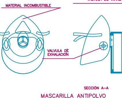
MASCARILLA ANTIPOLVO
