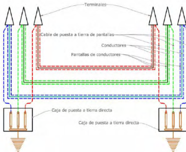
Figura 6.4. Esquema de conexión Solid Bonding
