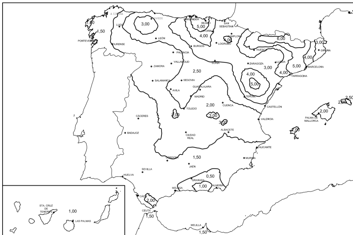
Figura 3.1. Mapa de densidad de impactos sobre el terreno N_g . [Fuente: Documento Básico SUA 8: Seguridad frente al riesgo causado por la acción del rayo.]
