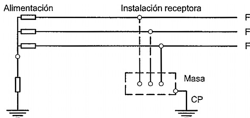
Figura 6.1. Esquema de distribución tipo IT
