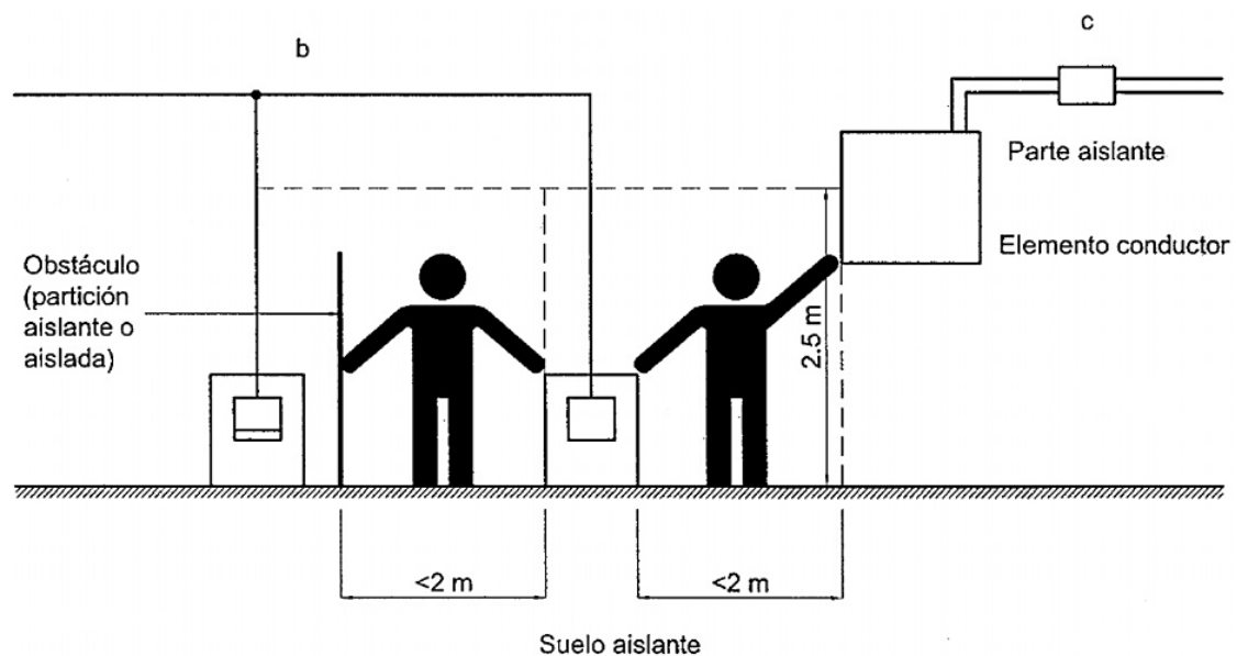
Figura 6.3. Esquema explicativo de los apartados b) y c)
