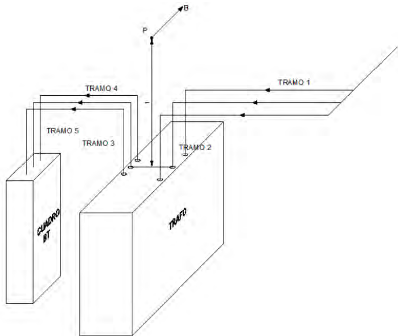
Figura 5.6. Cableado y trazado del transformador (simplificación)
