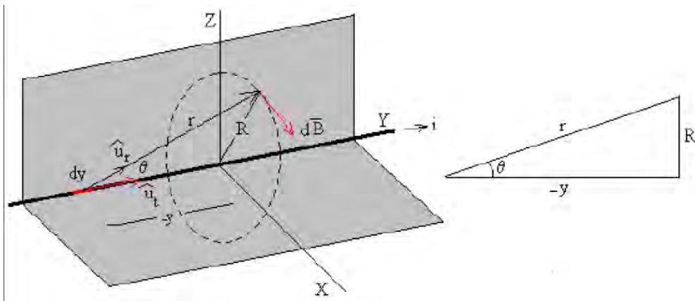
Figura 5.1. Cálculo del campo electromagnético generado por un conductor rectilíneo indefinido por el que circula una corriente i
