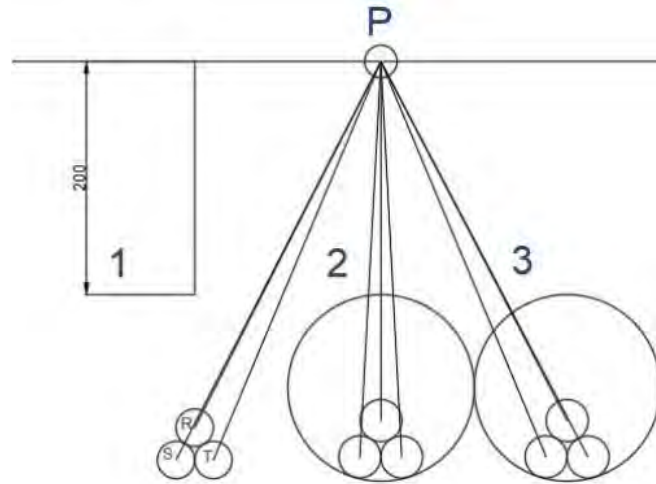
Figura 5.5. Punto P situado arriba de la terna de cables central
