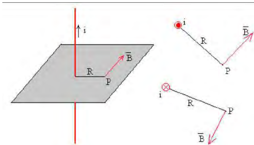
Figura 5.2. Campo magnético B, producido en el punto P
