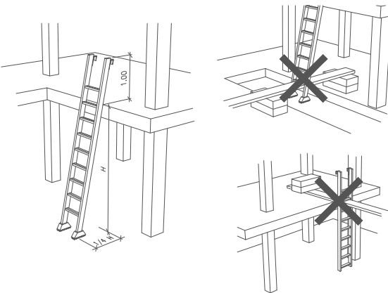
POSICION CORRECTA DE ESCALERAS DE MANO POSICIONES INCORRECTAS DE ESCALERAS DE MANO
