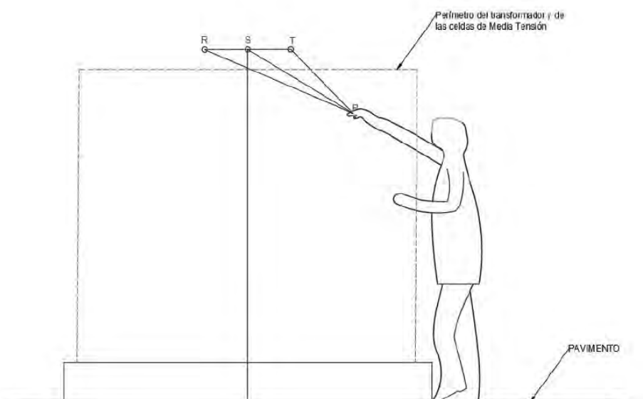
Figura 5.7. Esquema utilizado para la simulación
