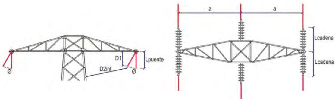
Ilustración 1: Apoyo n.º 1: Alineación-amarre
