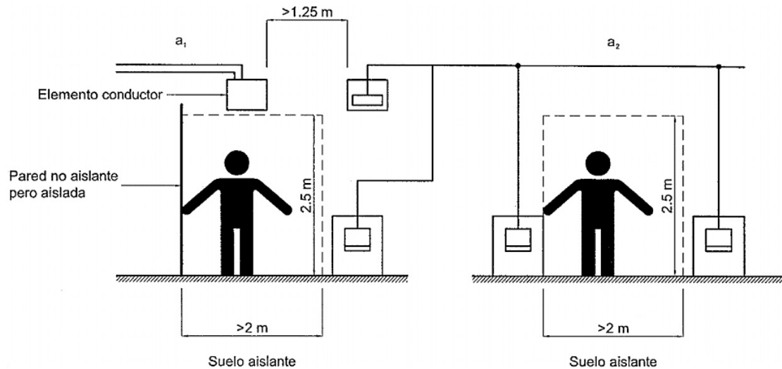
Figura 6.2. Esquema explicativo del apartado a)
