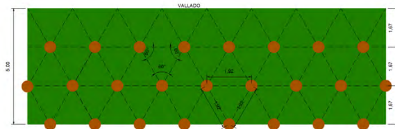
IMAGEN 1. ESQUEMA DEL MARCO DE PLANTACIÓN DE UNA ANCHURA DE 5 m
