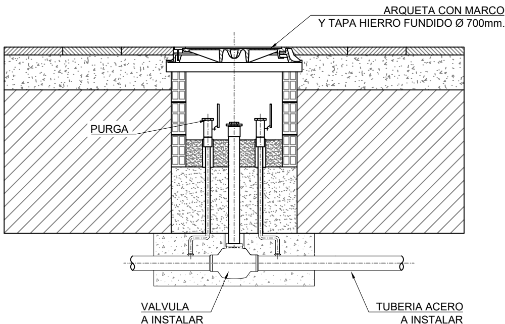
ALZADO
