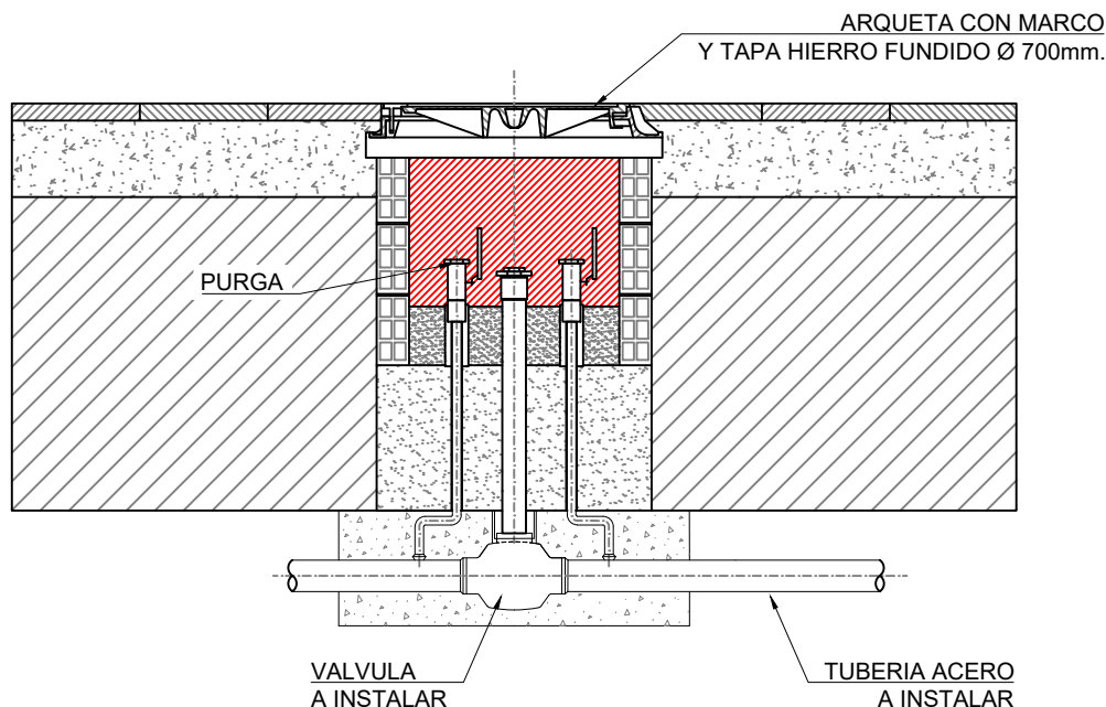
ALZADO
