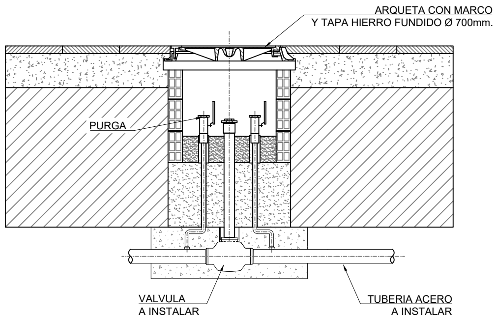
ALZADO
