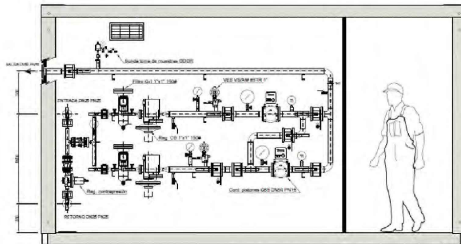
SECCION A-B
