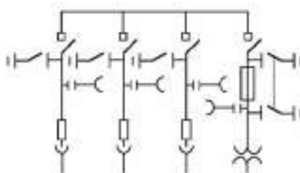
Fig. 11: Tres funciones de línea y una función de alimentación a servicios auxiliares
