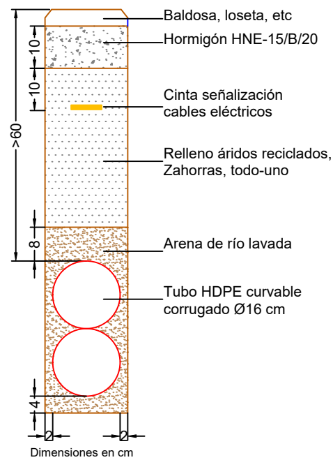
CANALIZACIÓN ENTUBADA 2T VERT. 160 EN ACERA/TIERRA ASIENTO ARENA
