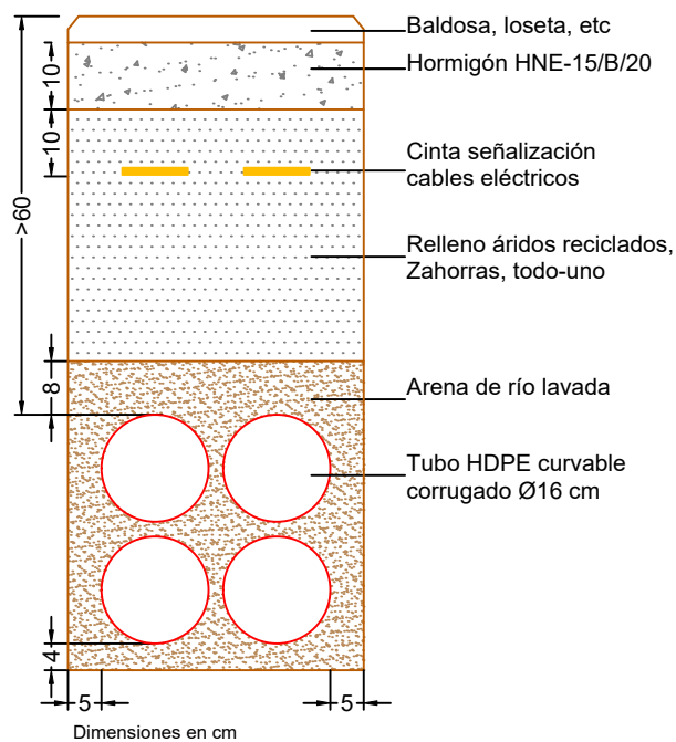
CANALIZACIÓN ENTUBADA 4T 160 EN ACERA/TIERRA ASIENTO ARENA
