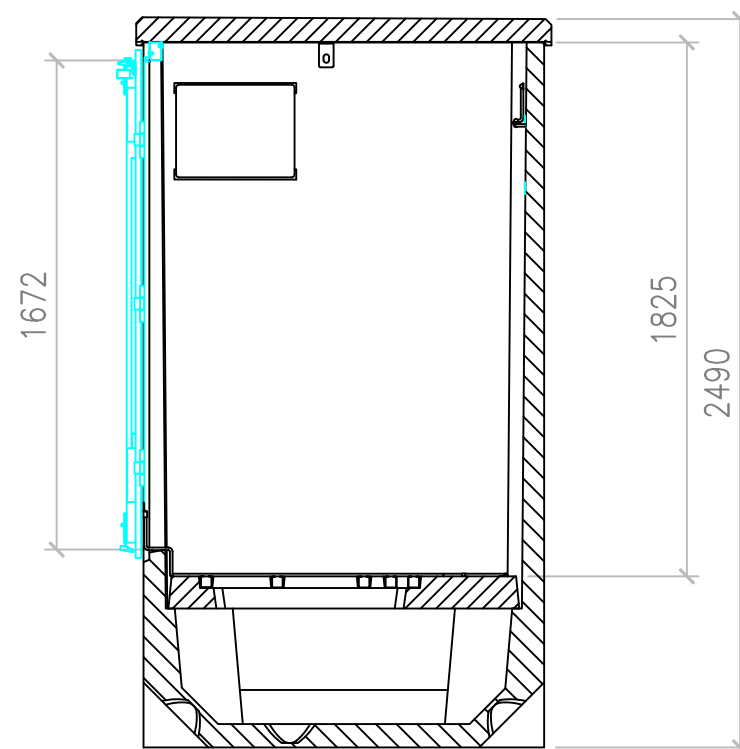
SECCIÓN A-A
