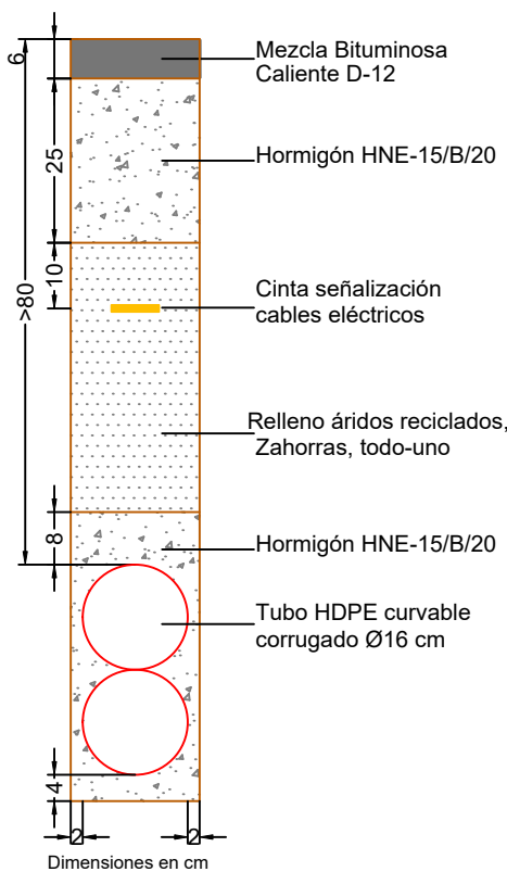
CANALIZACIÓN ENTUBADA 2T VERT. 160 EN CALZADA
