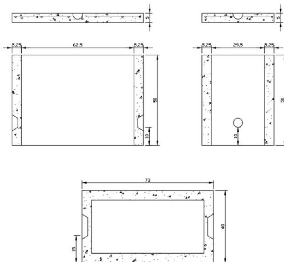
Figura 4. Arqueta
