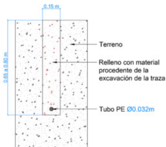
Figura 2. Esquema de microzanja
