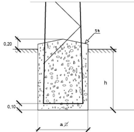
Cimentaciones para apoyos de perfiles metálicos
