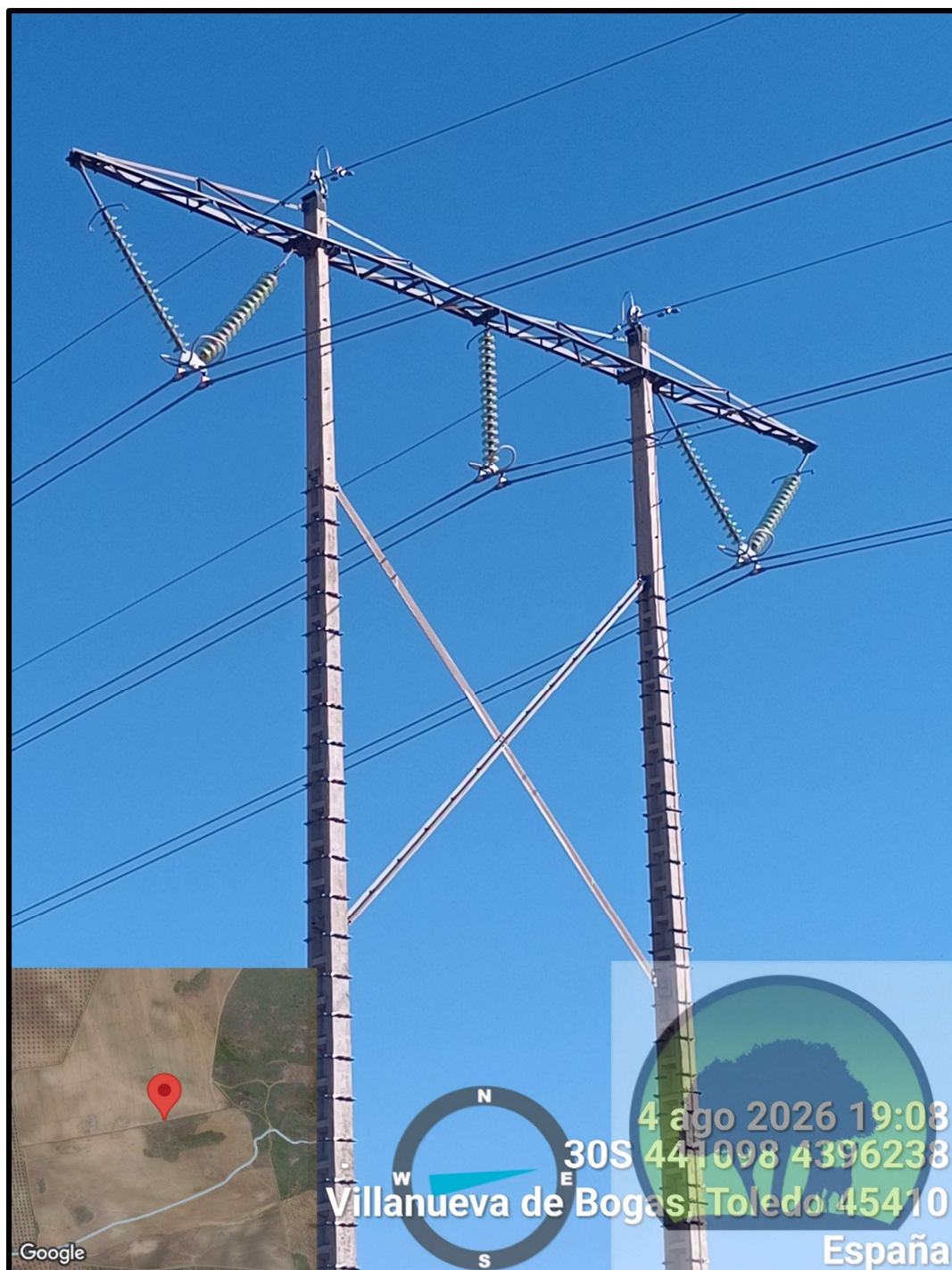
Foto 1: Apoyo tendido alta tensión.
