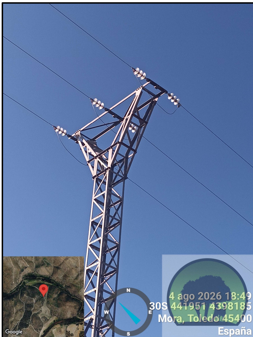
Foto 4: Apoyo bóveda, media tensión.
