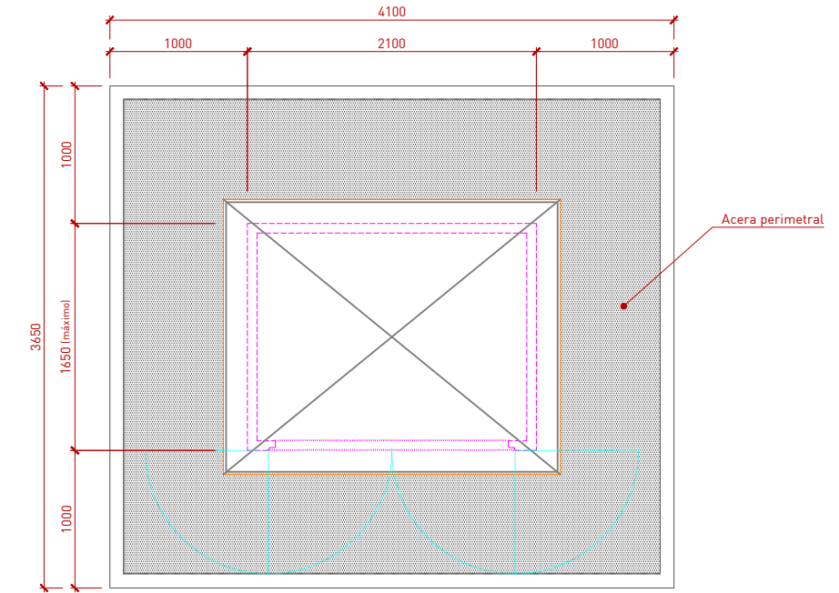
PLANTA EDIFICIO Y ACERA PERIMETRAL
